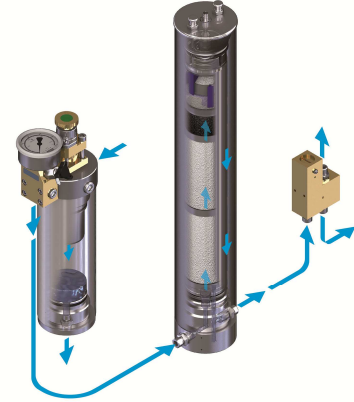
Filtersystem P41/350 (Abbildung ähnlich)
